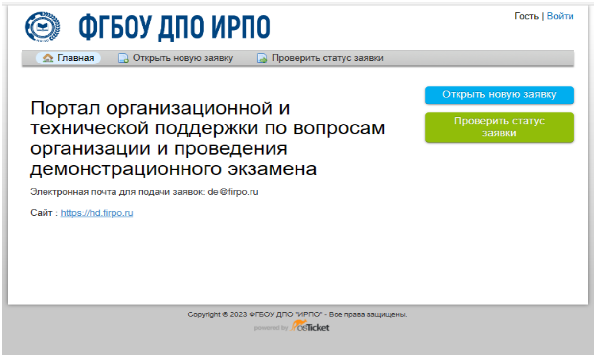
Рисунок 1 - Сайт регистрации
